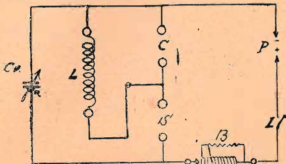
Fig. 1 - Schema elettrico
