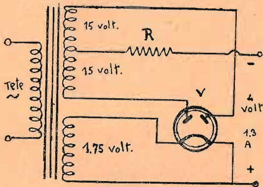
Schema elettrico
